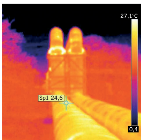
FOT. Obraz termowizyjny rur przesyłowych;
